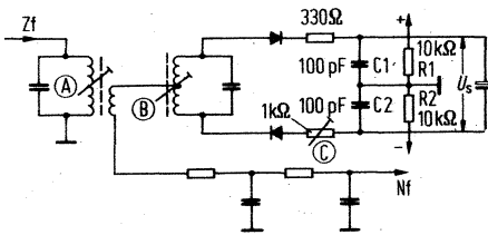
Bild 24. Grundschialtung des Ratiodektors
