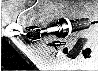
Aufshrumpfen eines Formteiles
