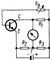
Bild 2. Prinzip der \beta -Bestimmung mit Brückenschaltung
