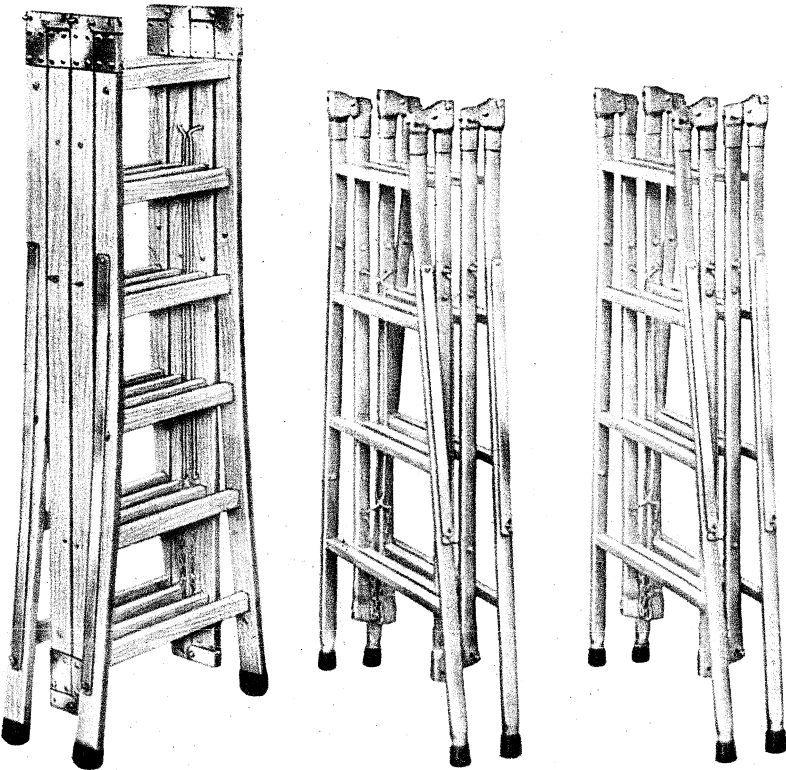
24d Schichtholz 6,20 m 24b Aluminium 4,80 m 24a Stahlrohr 4,22 m Funktion bei allen Modellen gleich. b Stahlrohr 4,80 m c Stahlrohr 6,00 m
