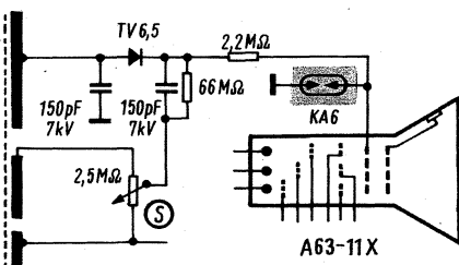
Durch Kriechstrom in der Fokus-Funkenstrecke bildete diese einen Nebenschluß, was die Fokusspannung verringerte
