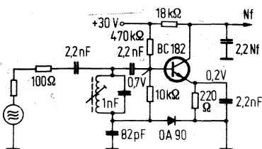
▲ Bild 21. Die Diodenstrecke D1 aus der vorhergehenden Schaltung ist durch die Emitter-Basisdiode eines Transistors ersetzt worden
