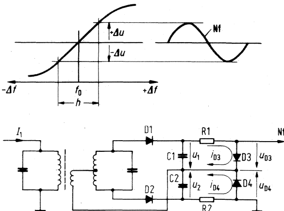
◀ Bild 15. Aus den Differenzspannungen der Diodengleichrichter ergibt sich die Umwandelkennlinie
