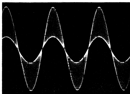
Bild 4. Oszillogramm des amplitudenmodulierten Tonsignals am Lautsprecher, über eine Modulationsperiode gespeichert. Zeitablenkung: 5 ms/Teil. Vertikalablenkung: 3 V/Teil. Frequenz: 50 Hz
