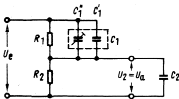
Bild 5.6. Frequenzkompensierter Spannungsteiler, Grundschaltung
