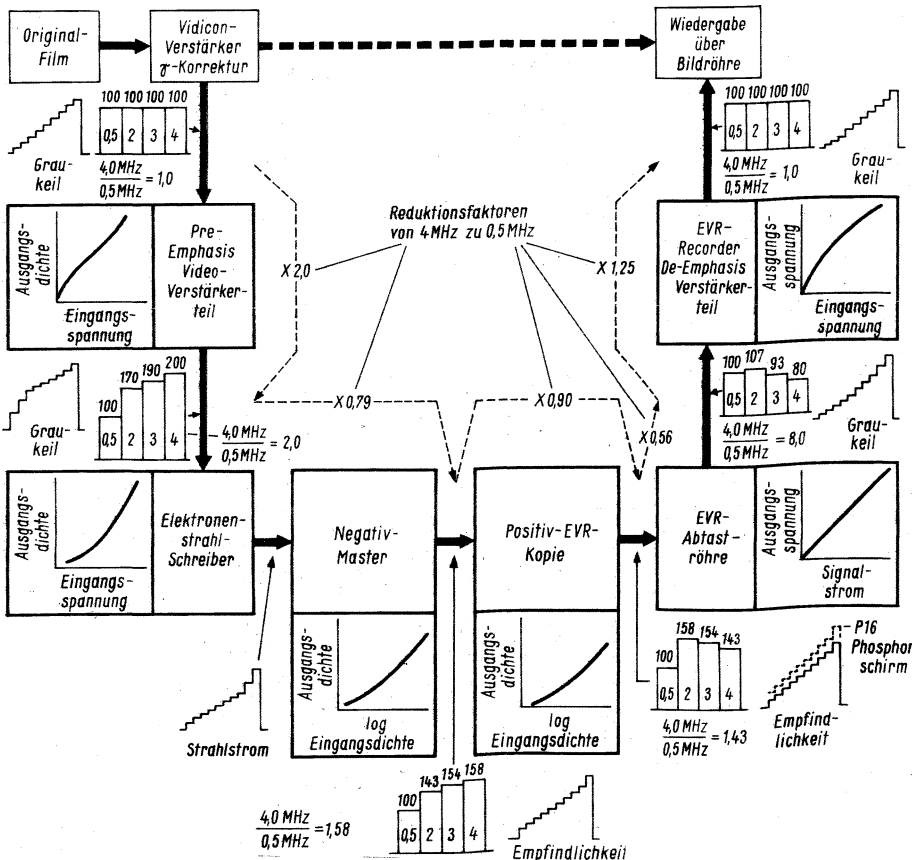
Bild 10. Amplituden-Frequenz-Charakteristiken sowie die zugehörigen Schwärzungsfunktionen innerhalb des EVR-Aufnahme- und Wiedergabesystems
