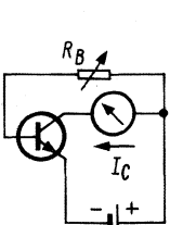
Bild 1. Prinzip der \beta -Bestimmung durch direkte Strommessung
